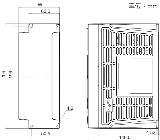
JSDAP-150A3/75B/100B 尺寸圖
