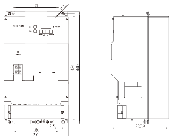
JSDAP-200A3/300A3 尺寸圖
